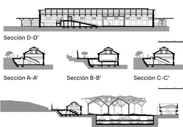
Sección Transversal General
